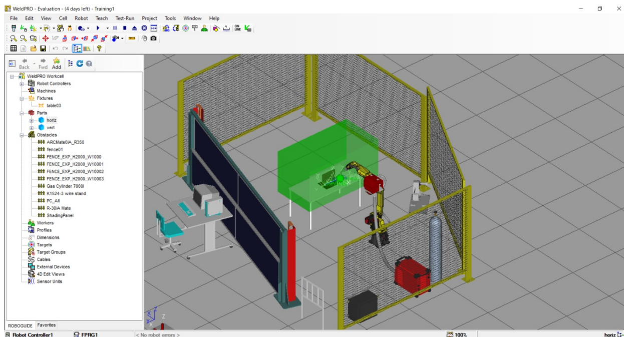
Модель роботизированной производственной ячейки в Roboguide
